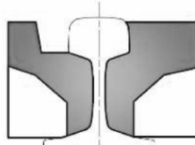
WERSJA 2 - "ETP" szyny: 49E1 (S49); płyta CBP rozstaw 670 mm
