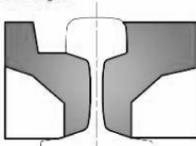
WERSJA 1 - "CBP" szyny: 49E1 (S49); płyta CBP rozstaw 600 mm
